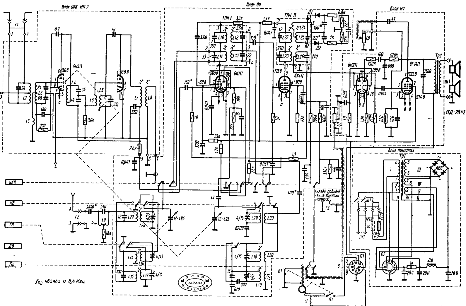
Принципиальная электрическая схема радиоприемника "Чайка-М"
