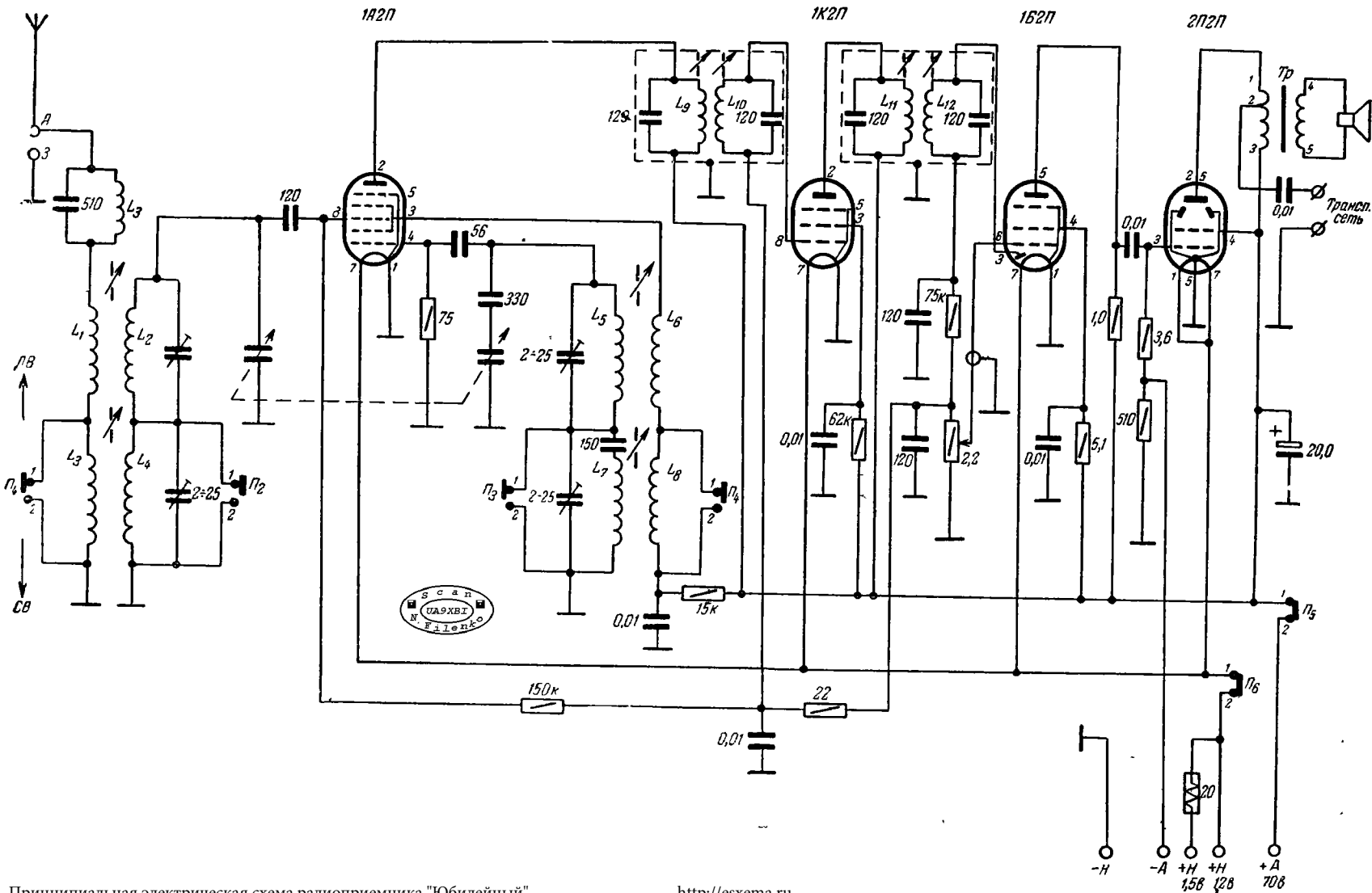
Принципиальная электрическая схема радиоприемника "Юбилейный"
