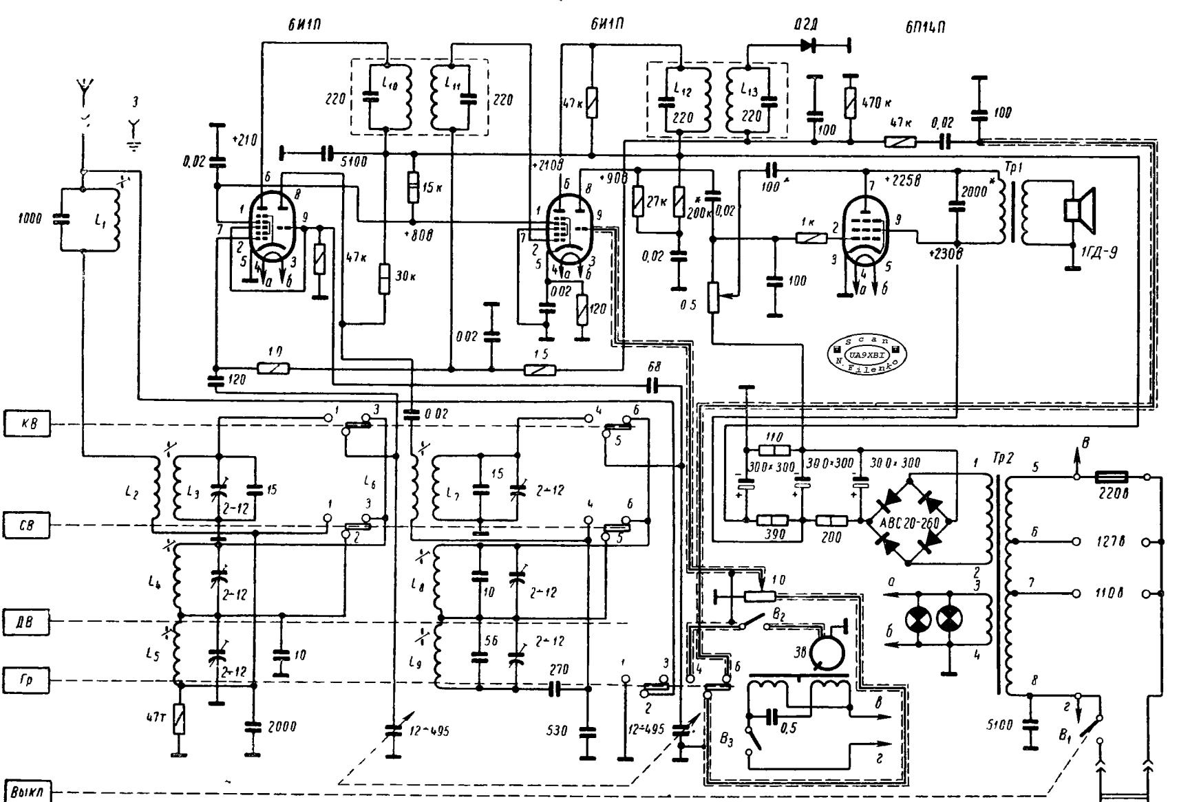
Принципиальная электрическая схема радиоприемника "Юность"
