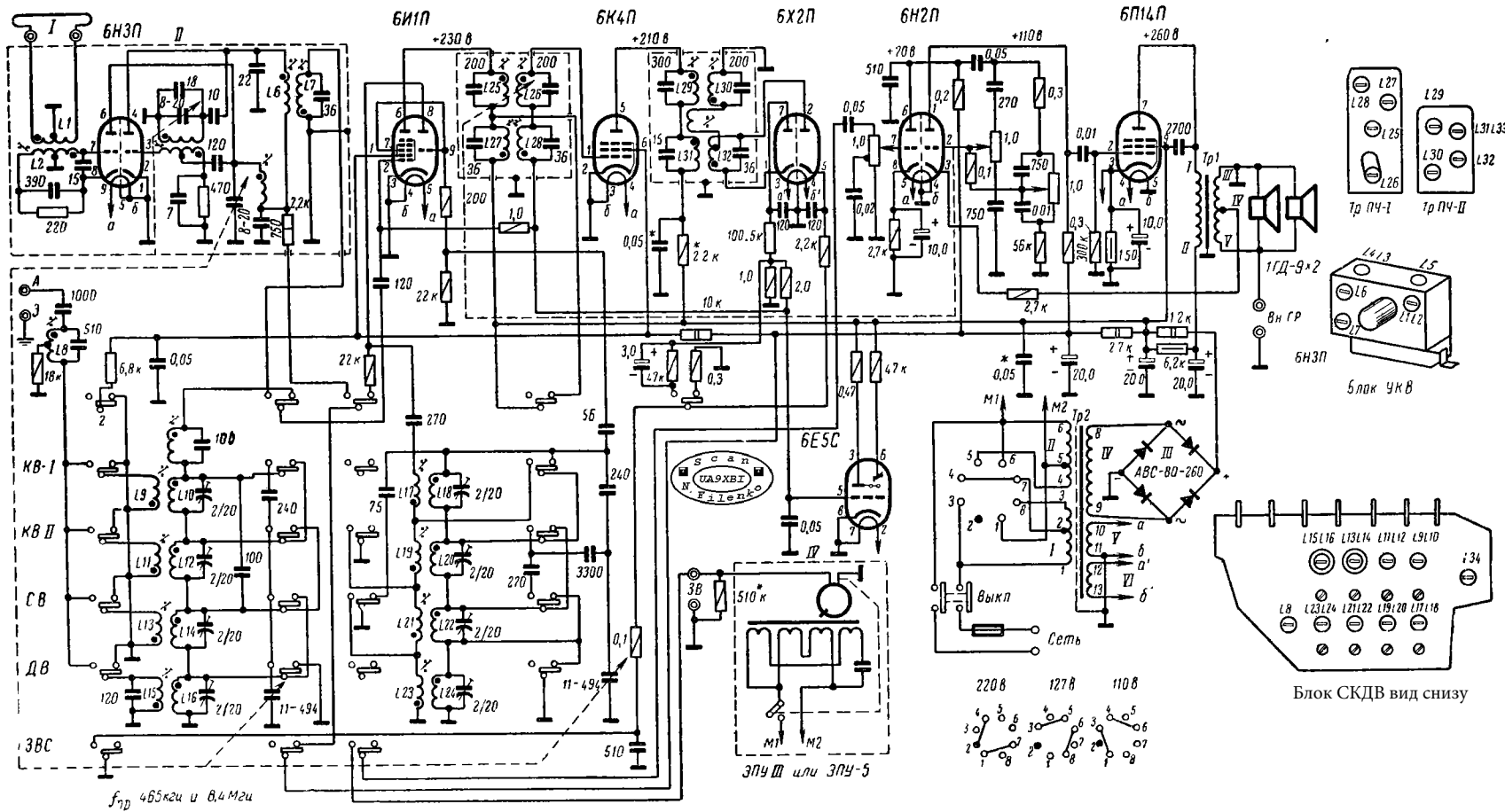
Принципиальная электрическая схема радиоприемника "Рассвет" I вариант
