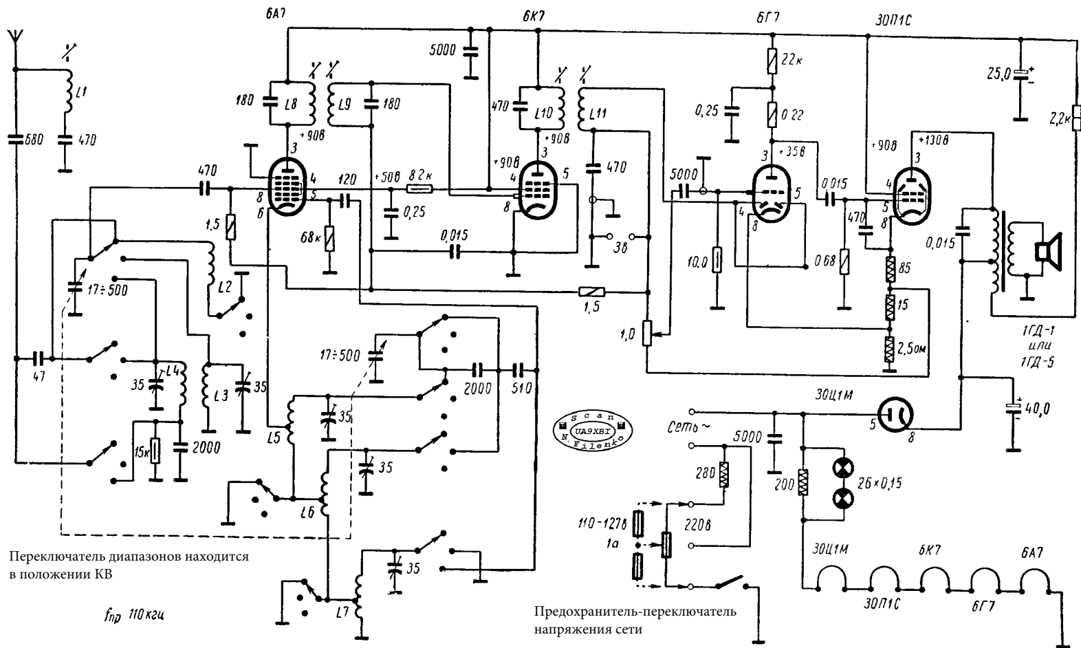
Принципиальная электрическая схема радиоприемника "Рекорд-47"
