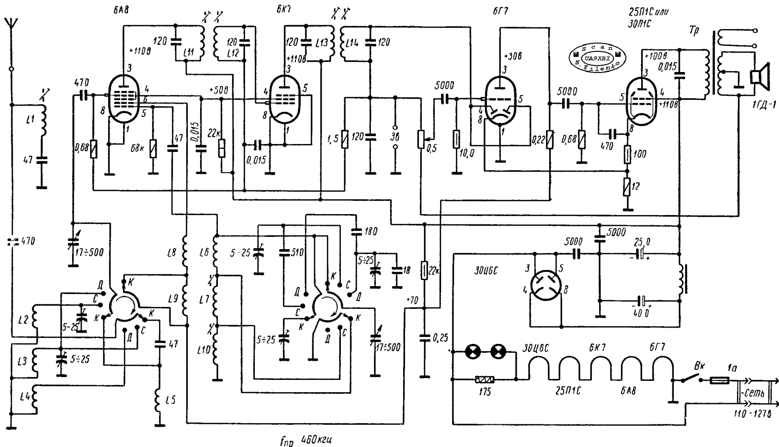
Принципиальная электрическая схема радиоприемника "Рекод"
