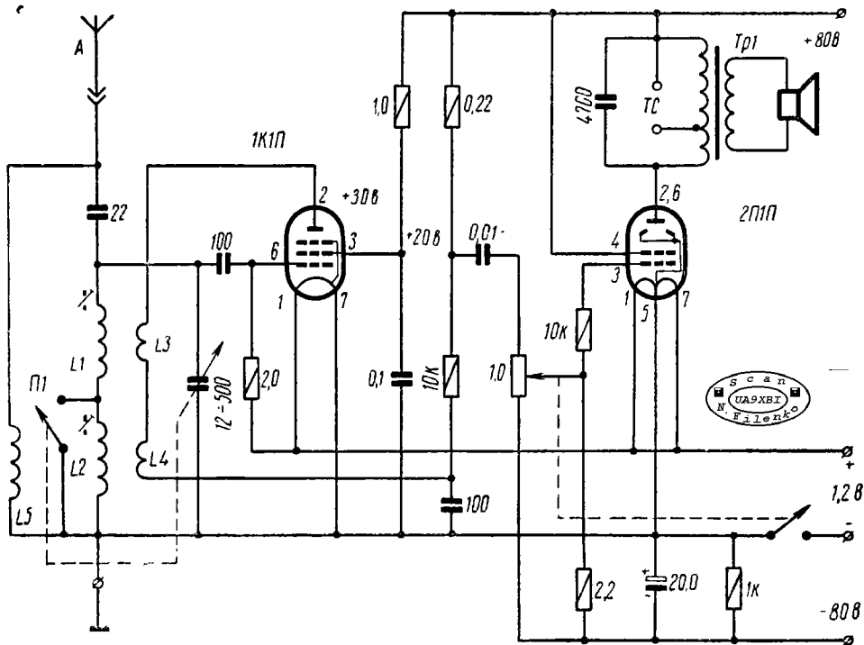
Принципиальная электрическая схема радиоприемника "Рига Б-912"
