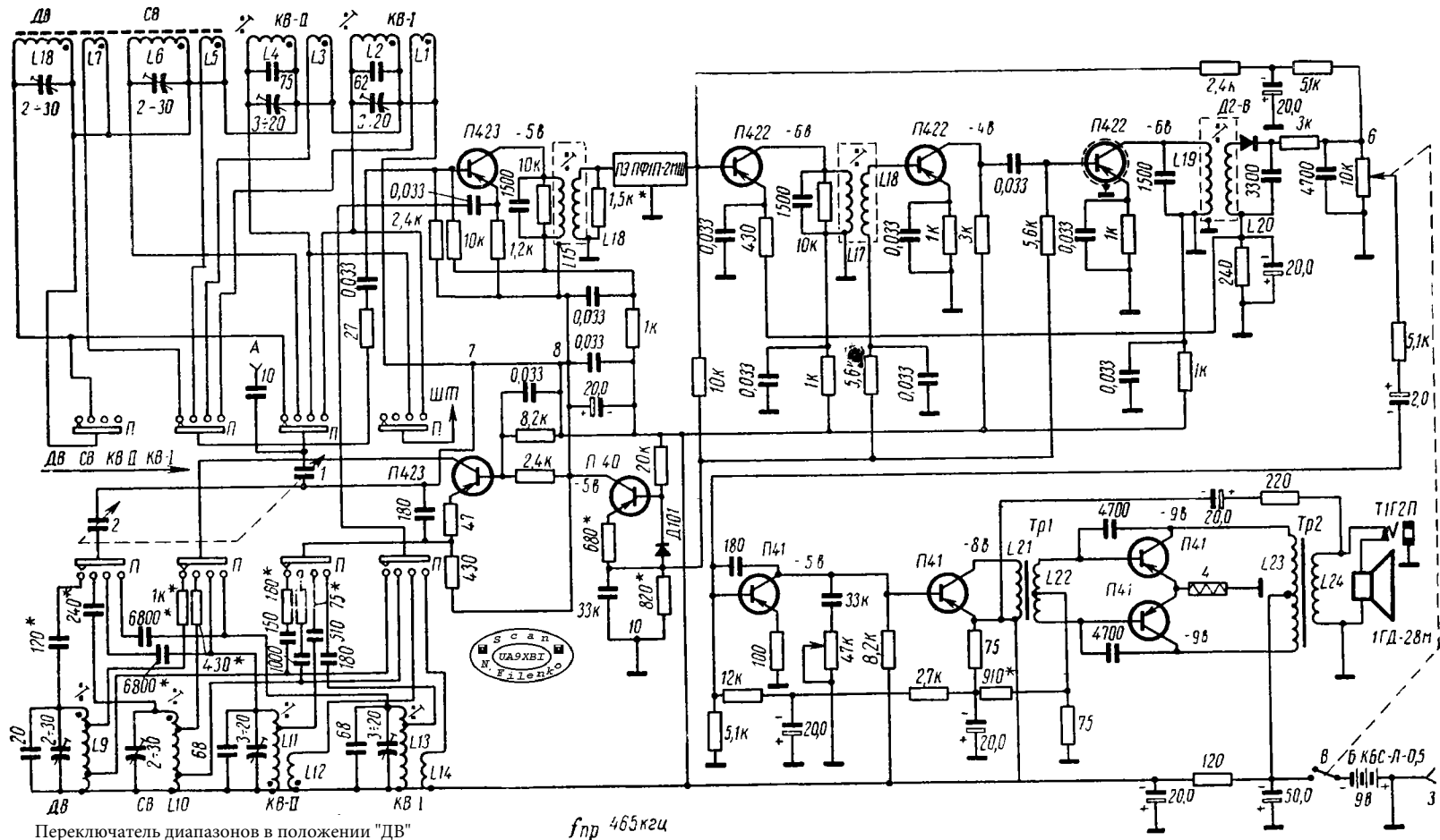
Принципиальная электрическая схема радиоприемника "Сувенир"
