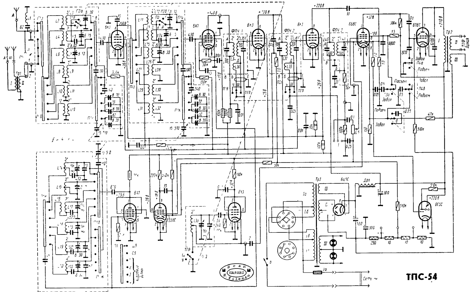
Принципиальная электрическая схема радиоприемника ТПС-54 http://esxema.ru/
