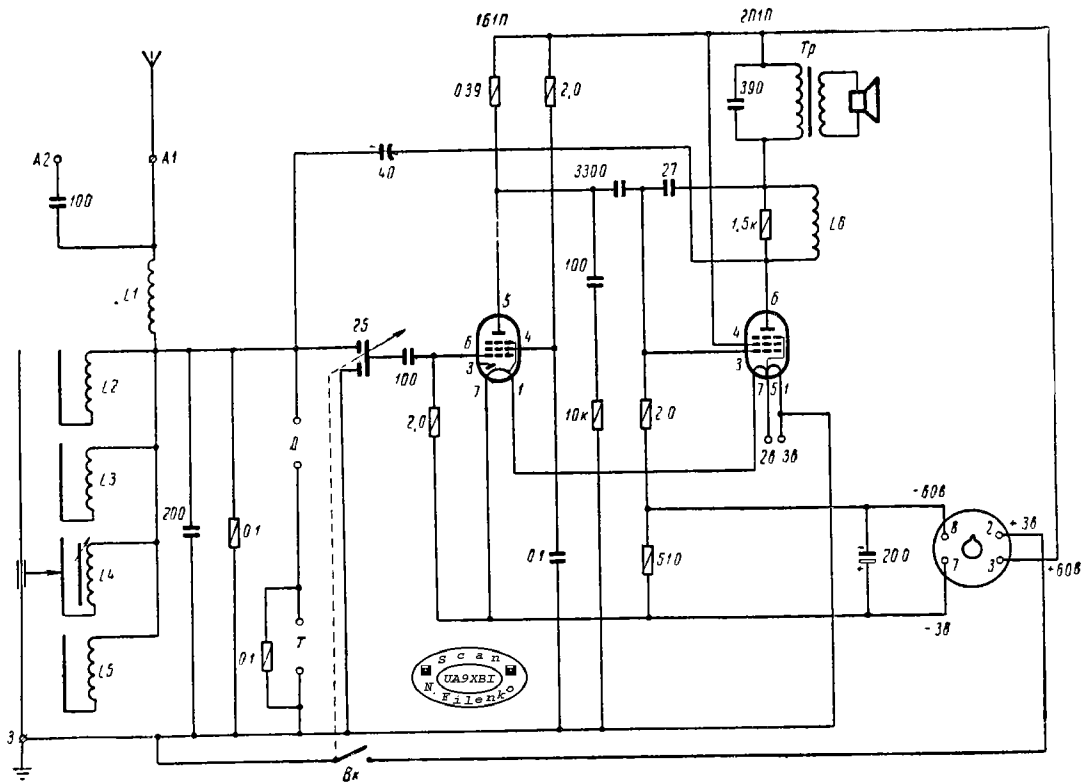
Электрическая принципиальная схема радиоприемника Тула http://esxema.ru/
