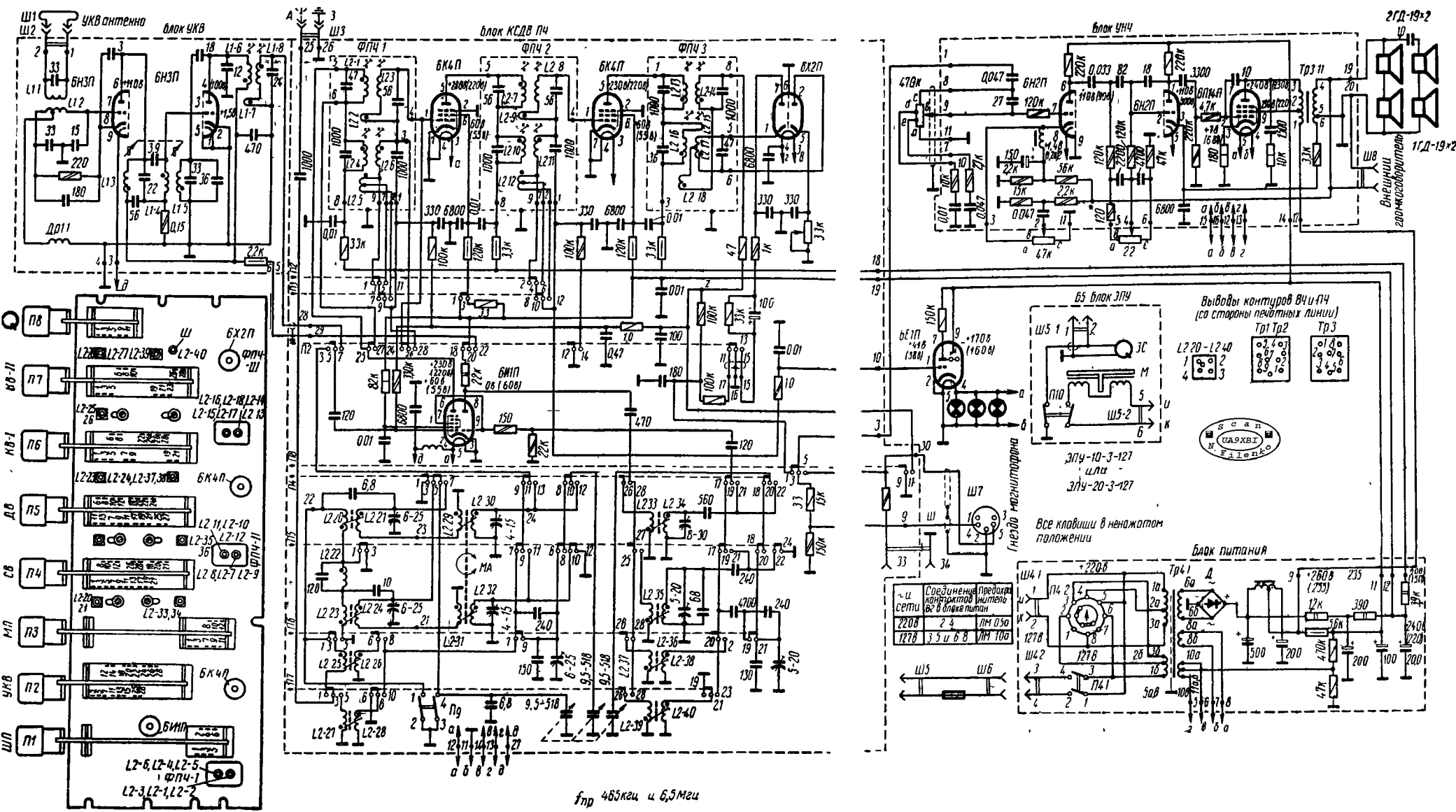
Принципиальная электрическая схема радиоприемника Урал-1 http://esxema.ru/
