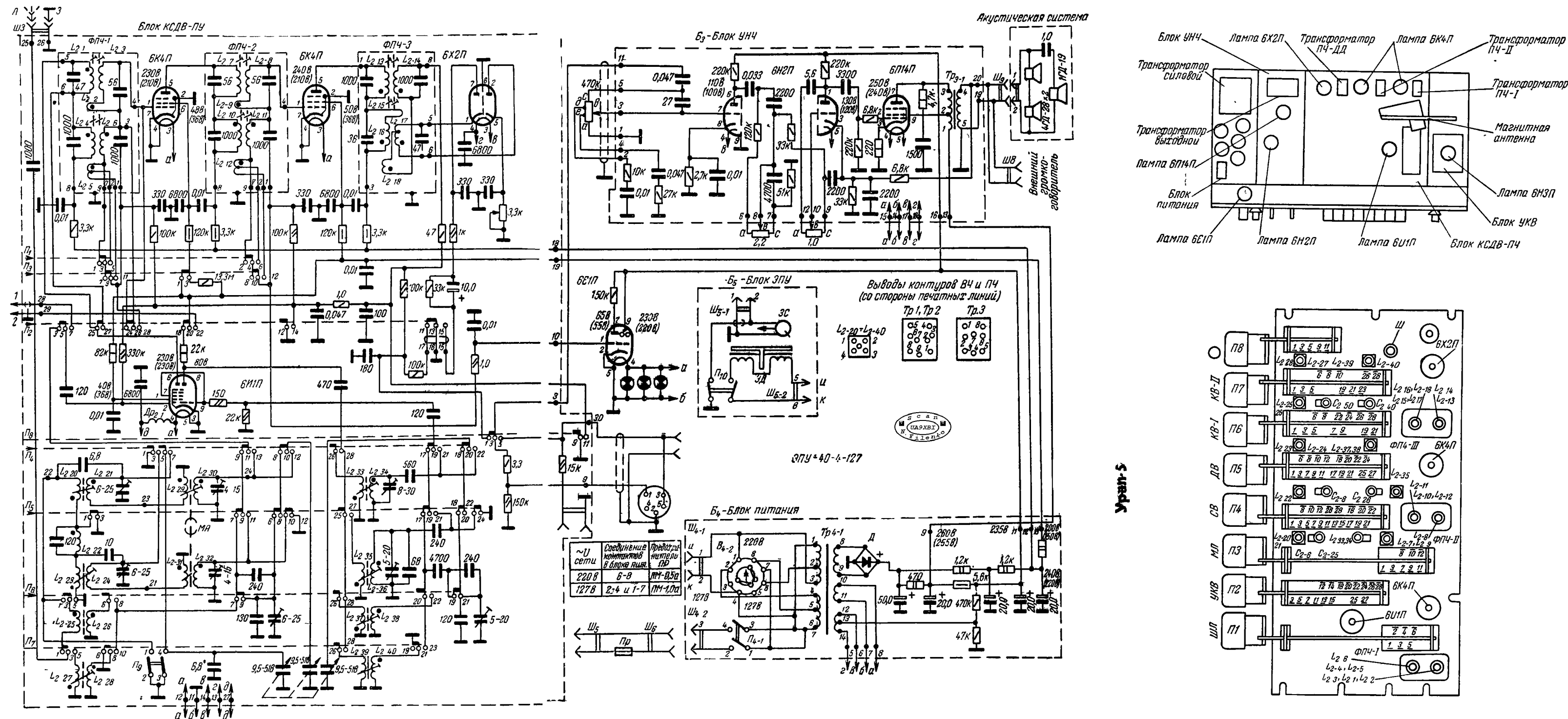
Принципиальная электрическая схема радиоприемника Урал-5 http://esxema.ru/
