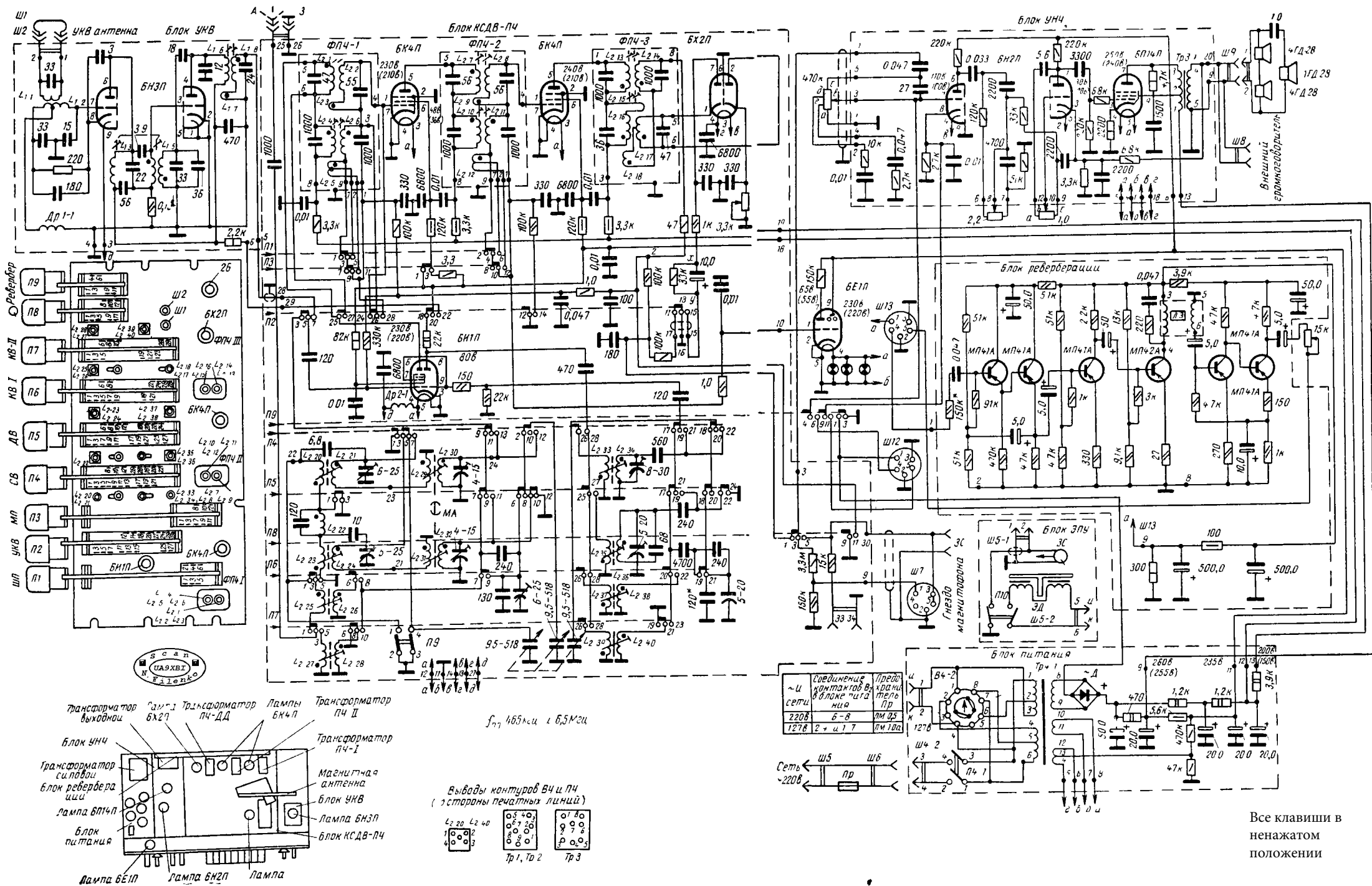
Принципиальная электрическая схема радиоприемника "Урал-7"
