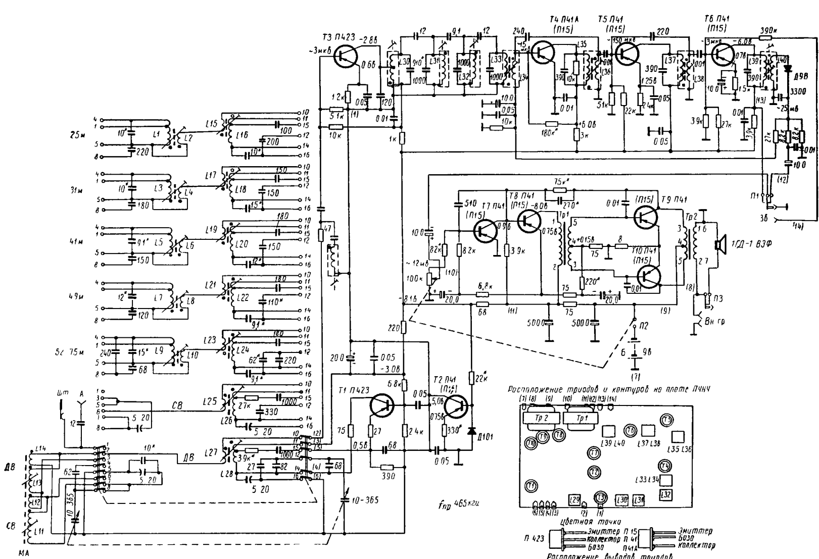
Принципиальная электрическая схема радиоприемника ВЭСпидола-10
