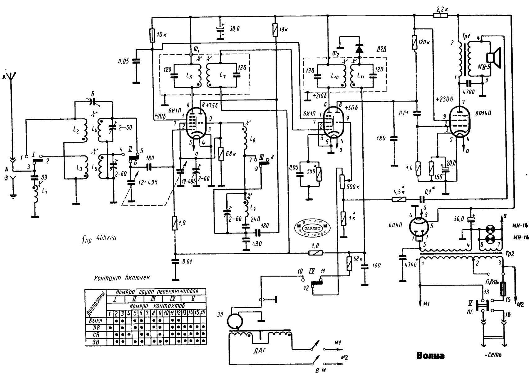
Принципиальная электрическая схема радиоприемника "Волна"
