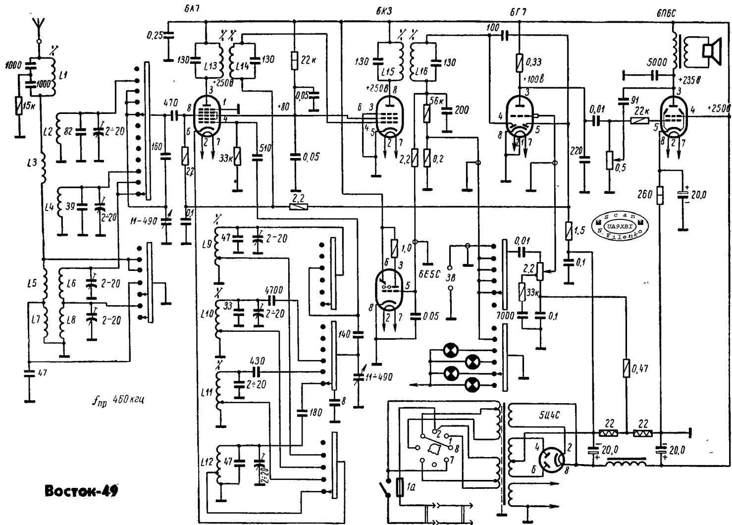
Принципиальная электрическая схема радиоприемника "Восток-49"
