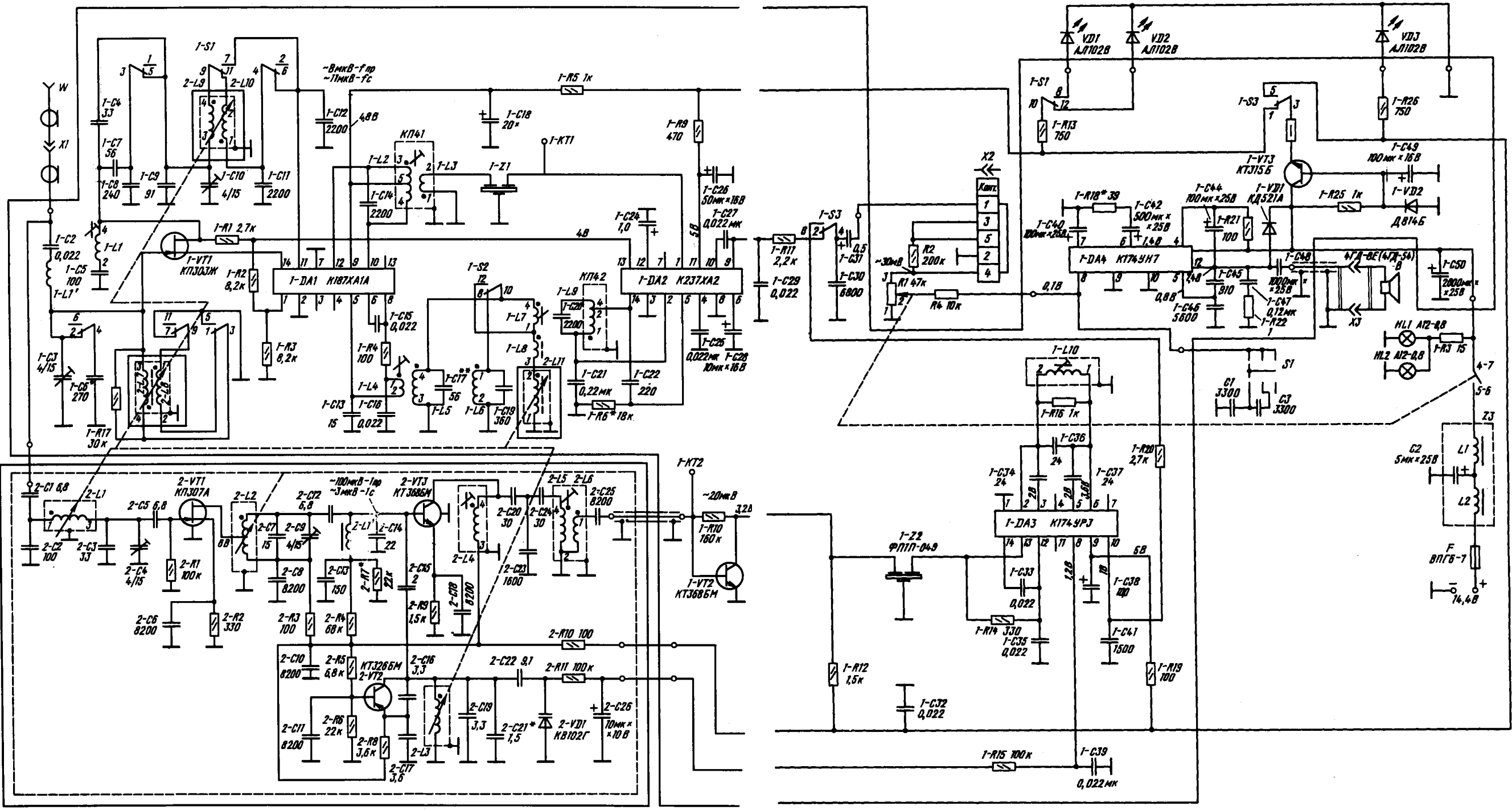
Принципиальная электрическая схема радиоприемника "Былина-207", "Былина-207В"
