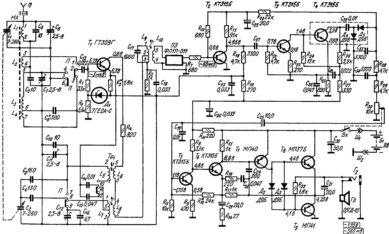
Принципиальная электрическая схема радиоприемника "Этюд-603
