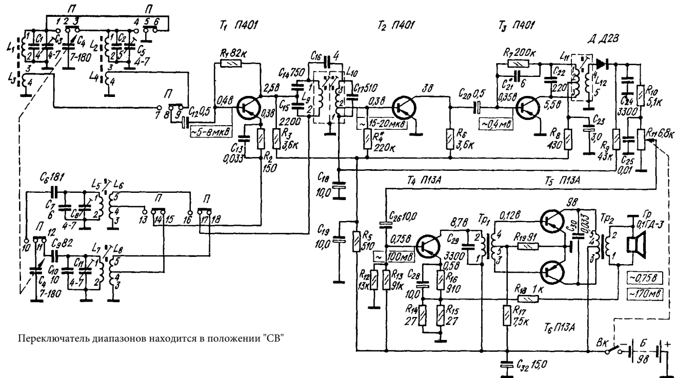
Принципиальная электрическая схема радиоприемника "Нева", "Чайка"
