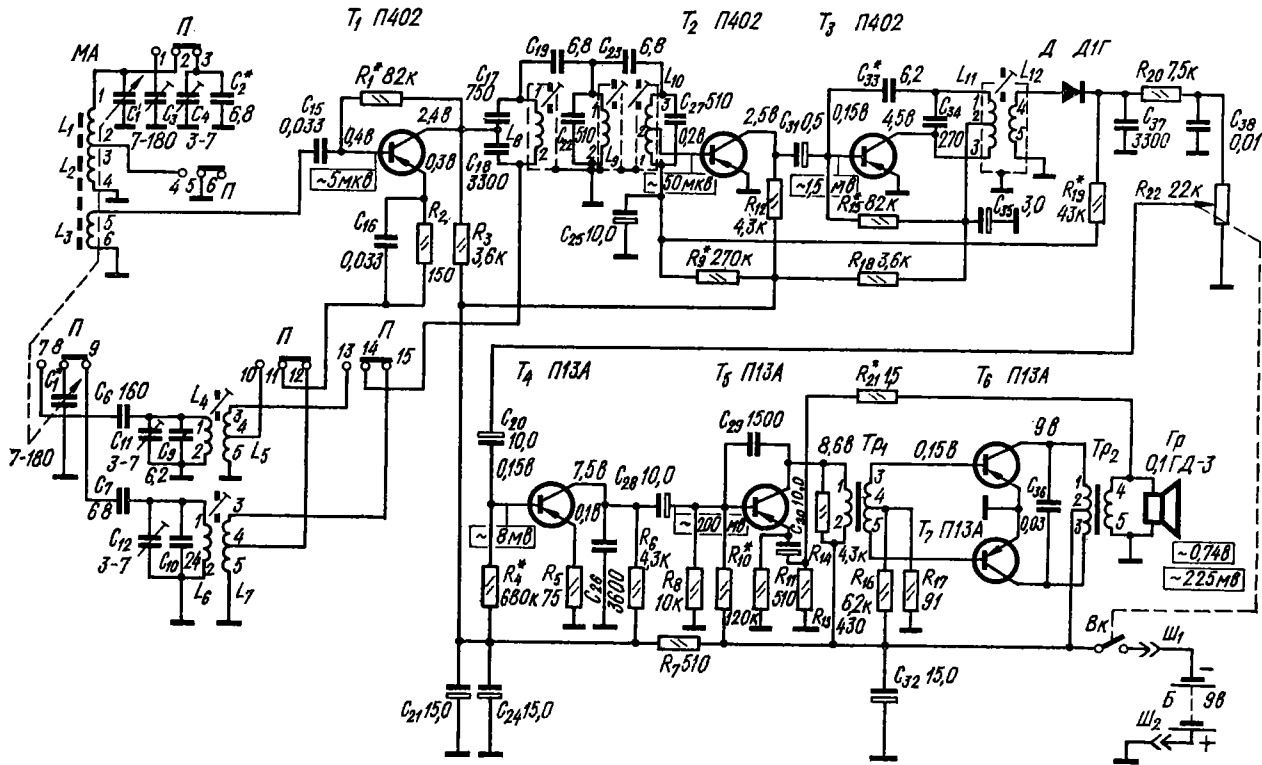
Принципиальная электрическая схема радиоприемника "Ласточка" http://esxema.ru/ (пе реключатель диапазонов в полож. ДВ)
