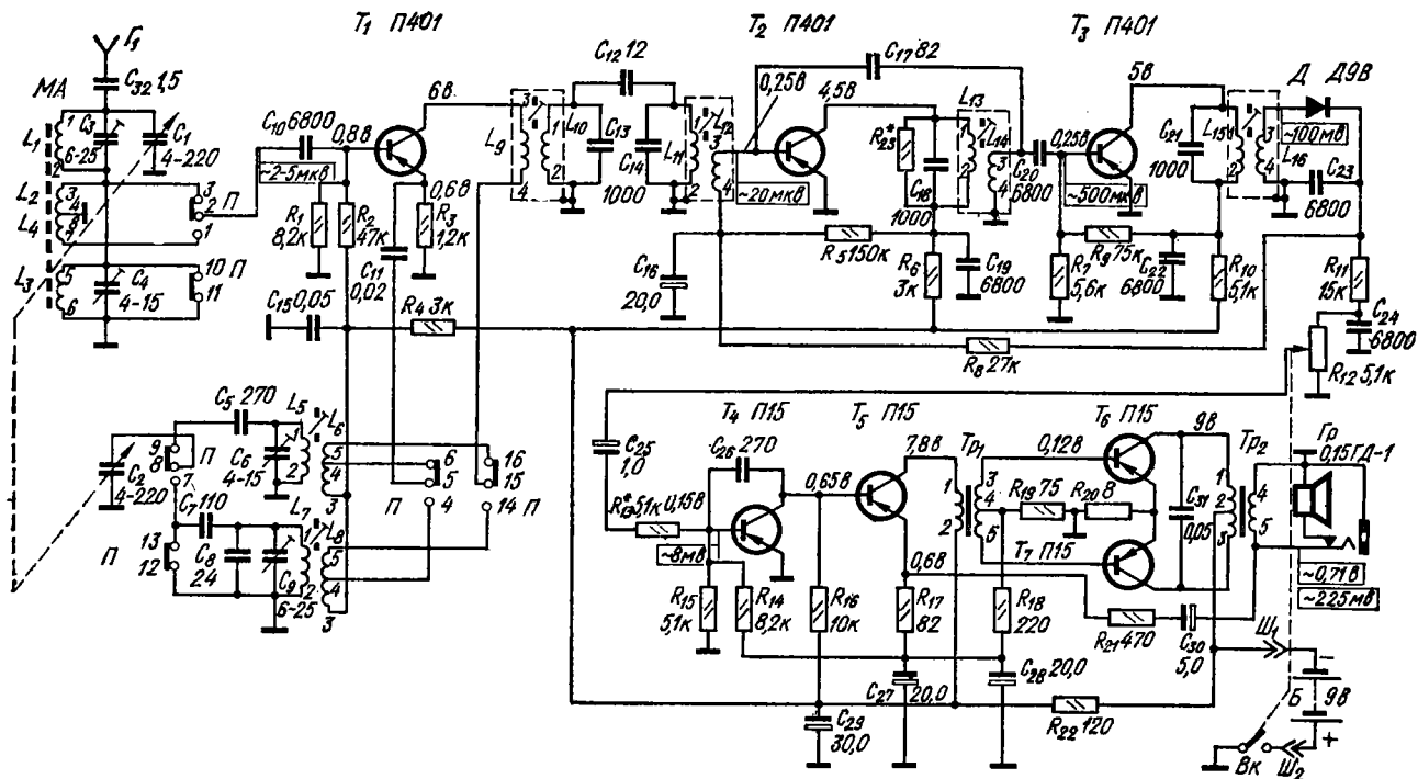
Принципиальная электрическая схема радиоприемника "Селга"
