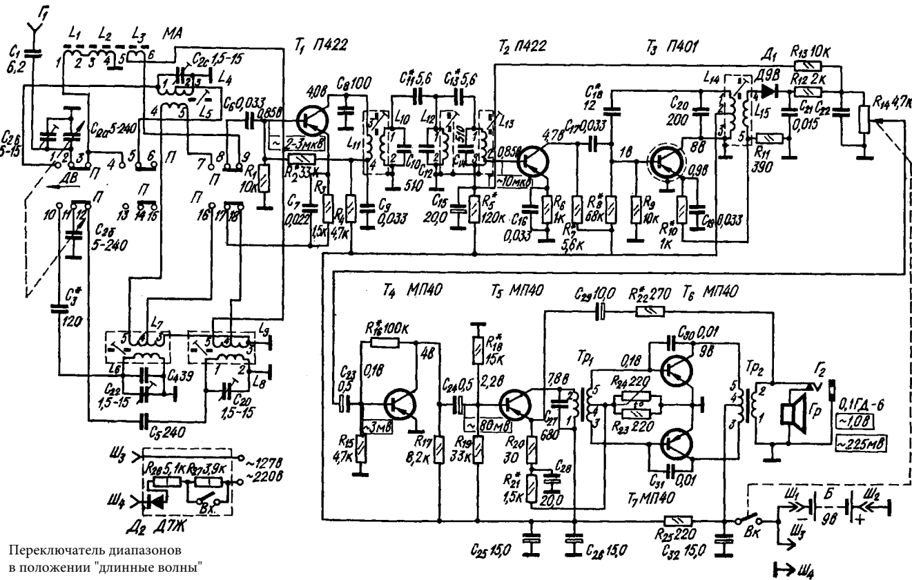
Принципиальная электрическая схема радиоприемника "Сокол", "Топаз-2", "Старт-2"
