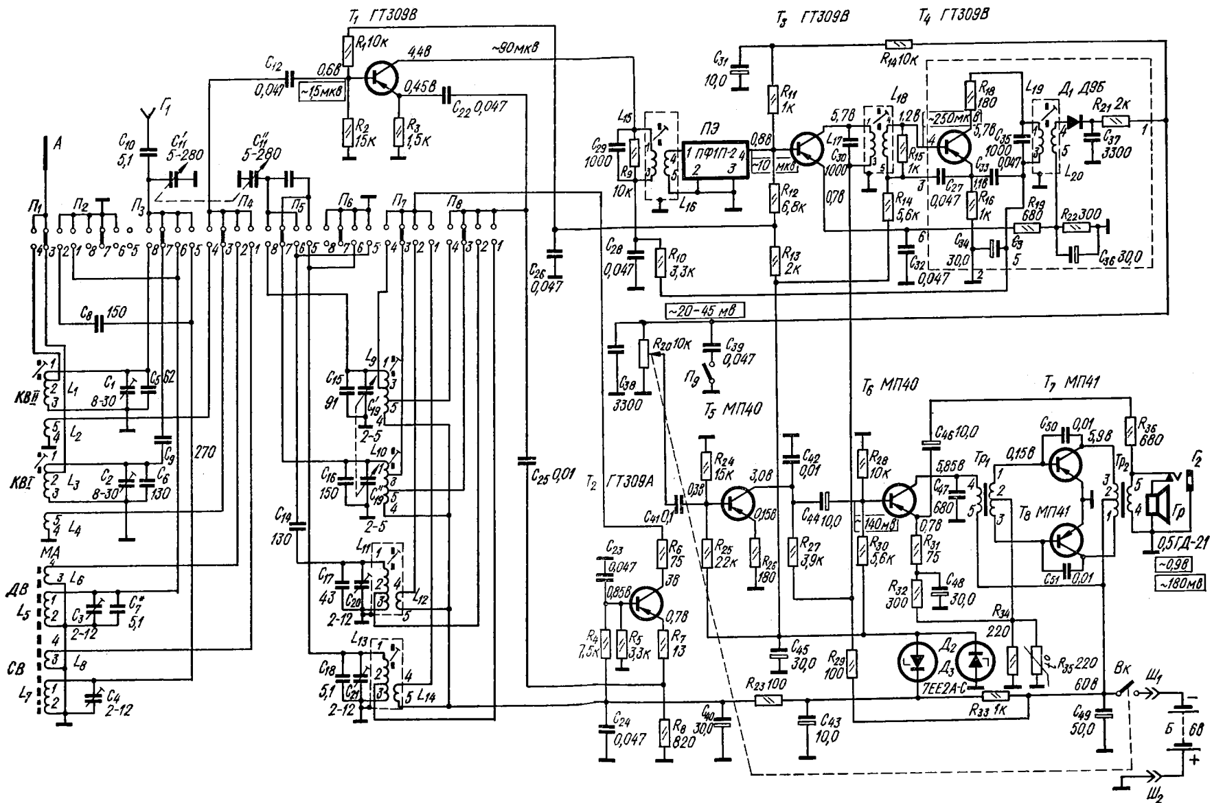
Принципиальная электрическая схема радиоприемника "Спорт 301"
