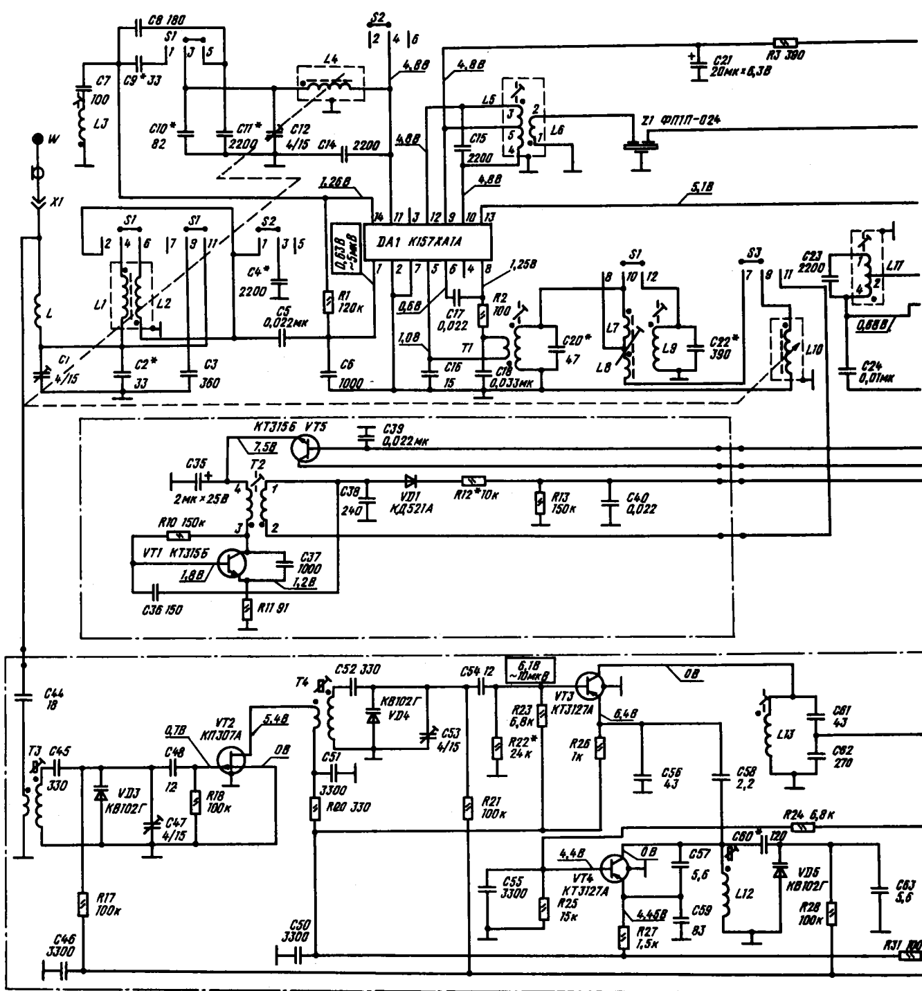
Принципиальная электрическая схема радиоприемника Тонар Авто-301 http://esxema.ru/
