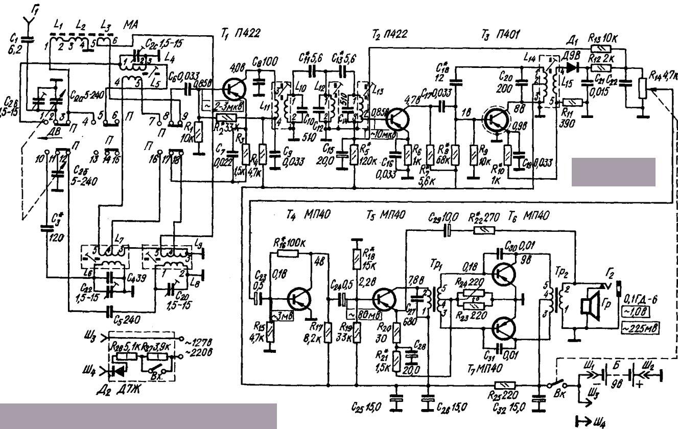
Принципиальная электрическая схема радиоприемников "Сокол", "Топаз-2", Старт-2" http://esxema.ru/
