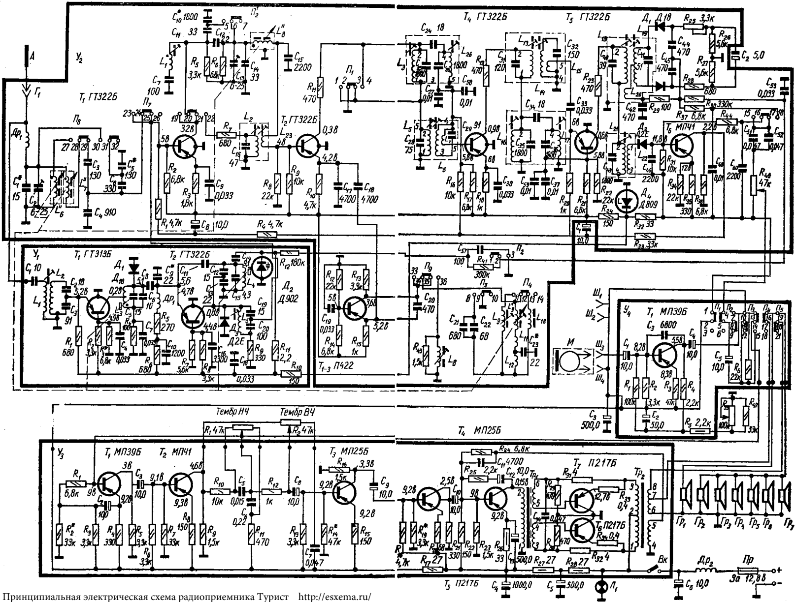
Принципиальная электрическая схема радиоприемника Турист http://esxema.ru/
