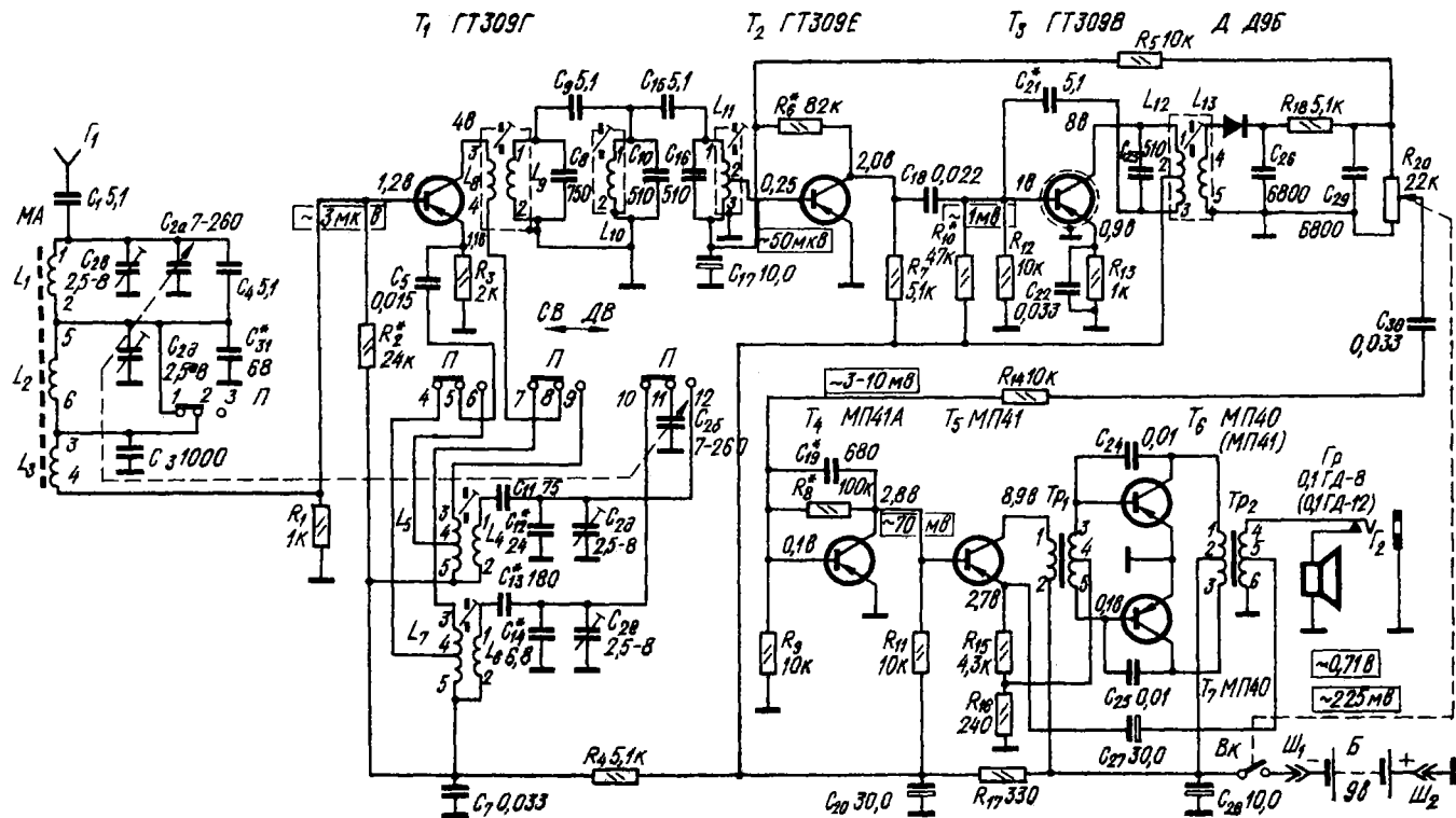
Принципиальная электрическая схема радиоприемника "Юпитер-601", "Юпитер-М"
