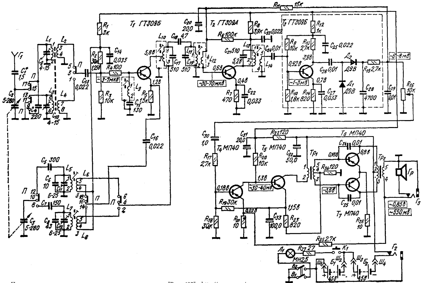
Принципиальная электрическая схема радиоприемника "Beta-402" http://esxema.ru/
