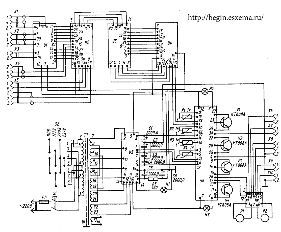
Схема электрическая принципиальная Электрофона «Актур-003» стерео
