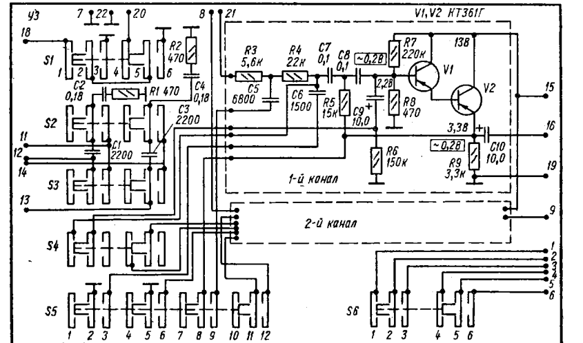
Схема электрическая принципиальная Электрофона «Актур-003» стерео
