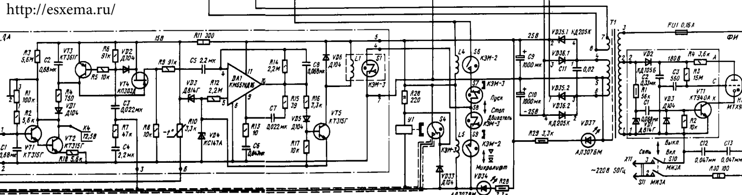
Электрическая схема принципиальная электропроигрывателя «Корвет-38» стерео
