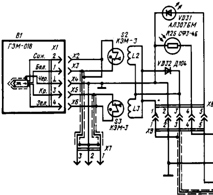
Электрическая схема принципиальная электропроигрывателя «Корвет-38» стерео
