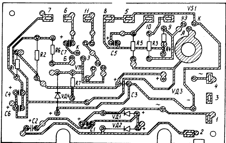
Электромонтажный чертеж печатной платы
