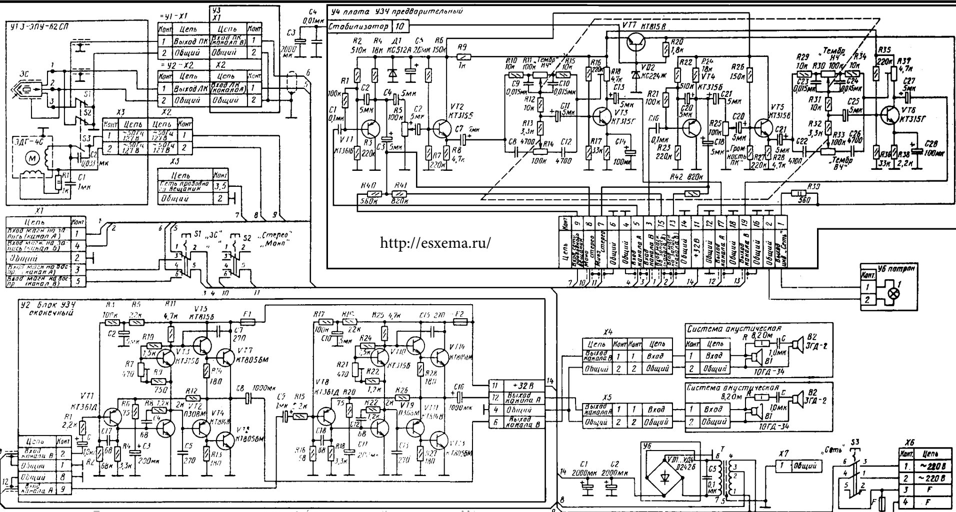
Принципиальная схема электрофона «Радиотехника 301» - стерео
