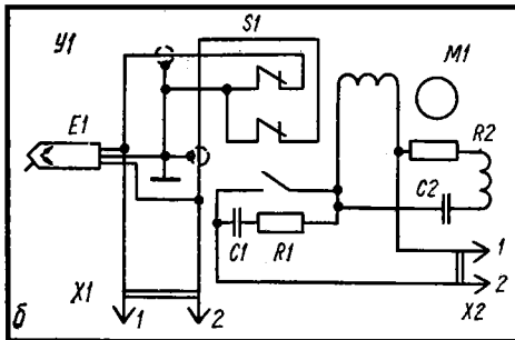
Принципиальная схема электрофона «Рондо-204» - стерео, «Рондо-203»
