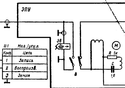
Схема электрическая принципиальная электрофона «Аккорд-202» стерео Переклюатель установлен в позицию «электрофон»
