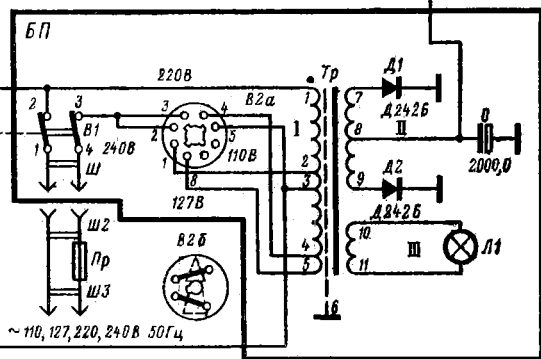
Схема электрическая принципиальная электрофона «Аккорд-202» стерео Переклюатель установлен в позицию «электрофон»
