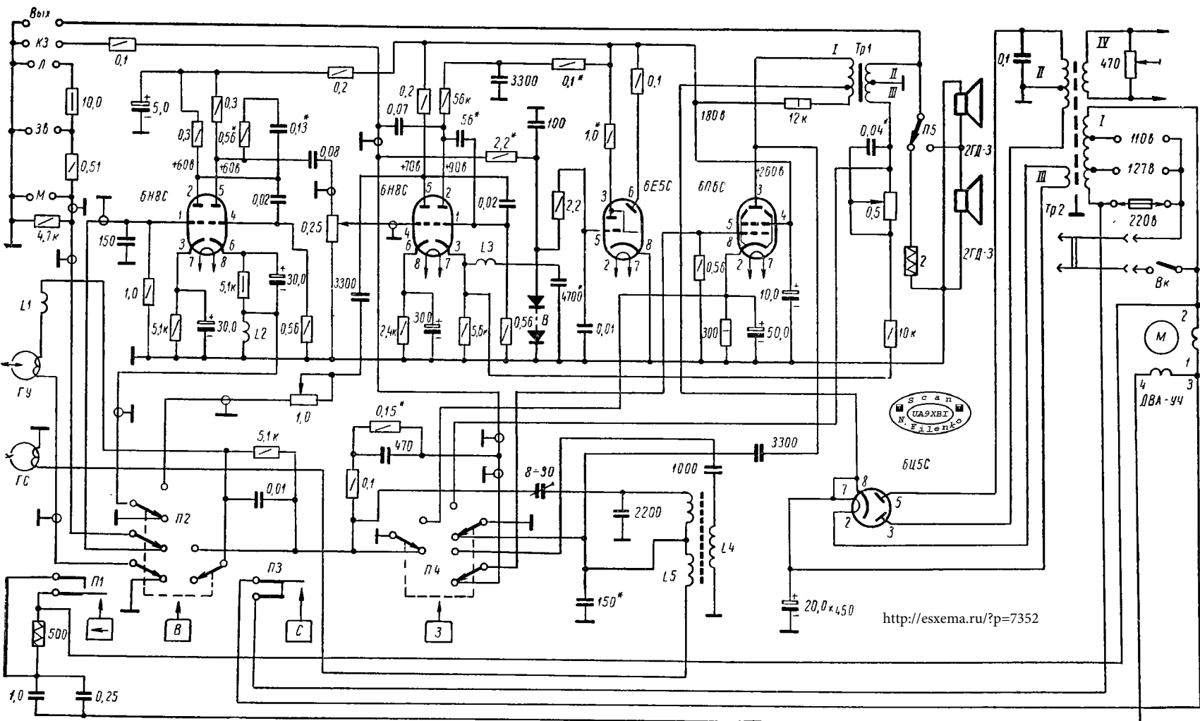
Принципиальная электрическая схема магнитофона «Днепр-9»
