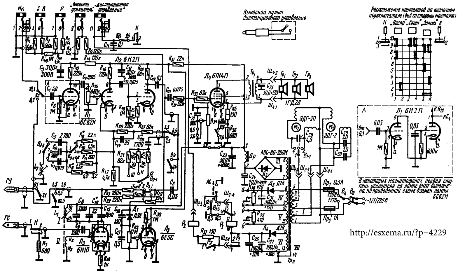
Принципиальная электрическая схема магнитофона «Комета МГ-201» в режиме Запись при скорости ленты 19.09 см/сек (выпуск 1968 г)
