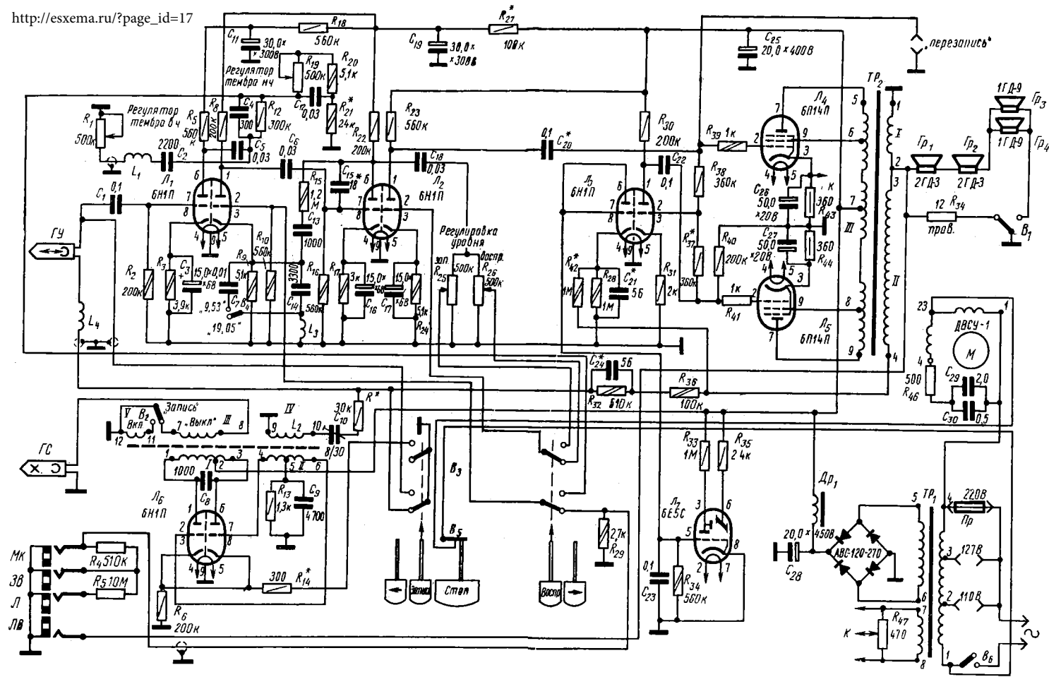
Принципиальная электрическая схема магнитофона «Днепр-11» в режиме «Стоп» при скорости 19.05 см/с
