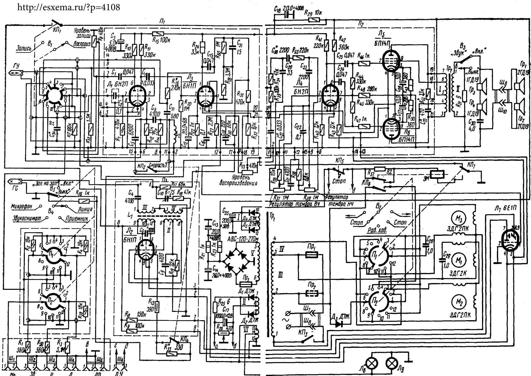
Принципиальная электрическая схема магнитофона «Днепр 14-А»
