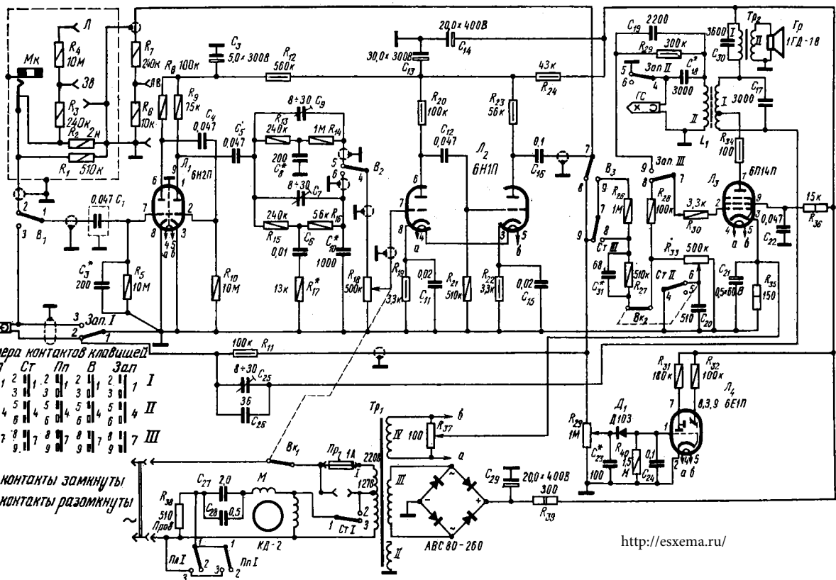
Принципиальная электрическая схема магнитофона «Айда» в режиме «СТОП» (выпуск до 1965 г.)
