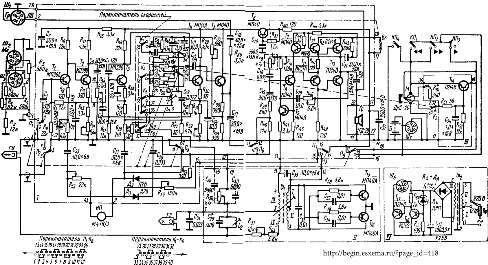
Принципиальная электрическая схема магнитофона «Романтик-3» в режиме Воспроизведение при скорости 9.53 см/с
