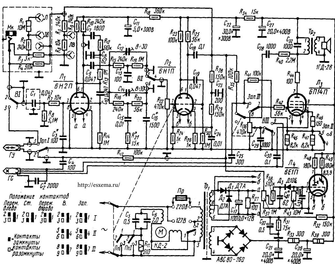
Принципиальная электрическая схема магнитофона «Айдаc» в режиме «СТОП» (выпуск после 1965 г.)
