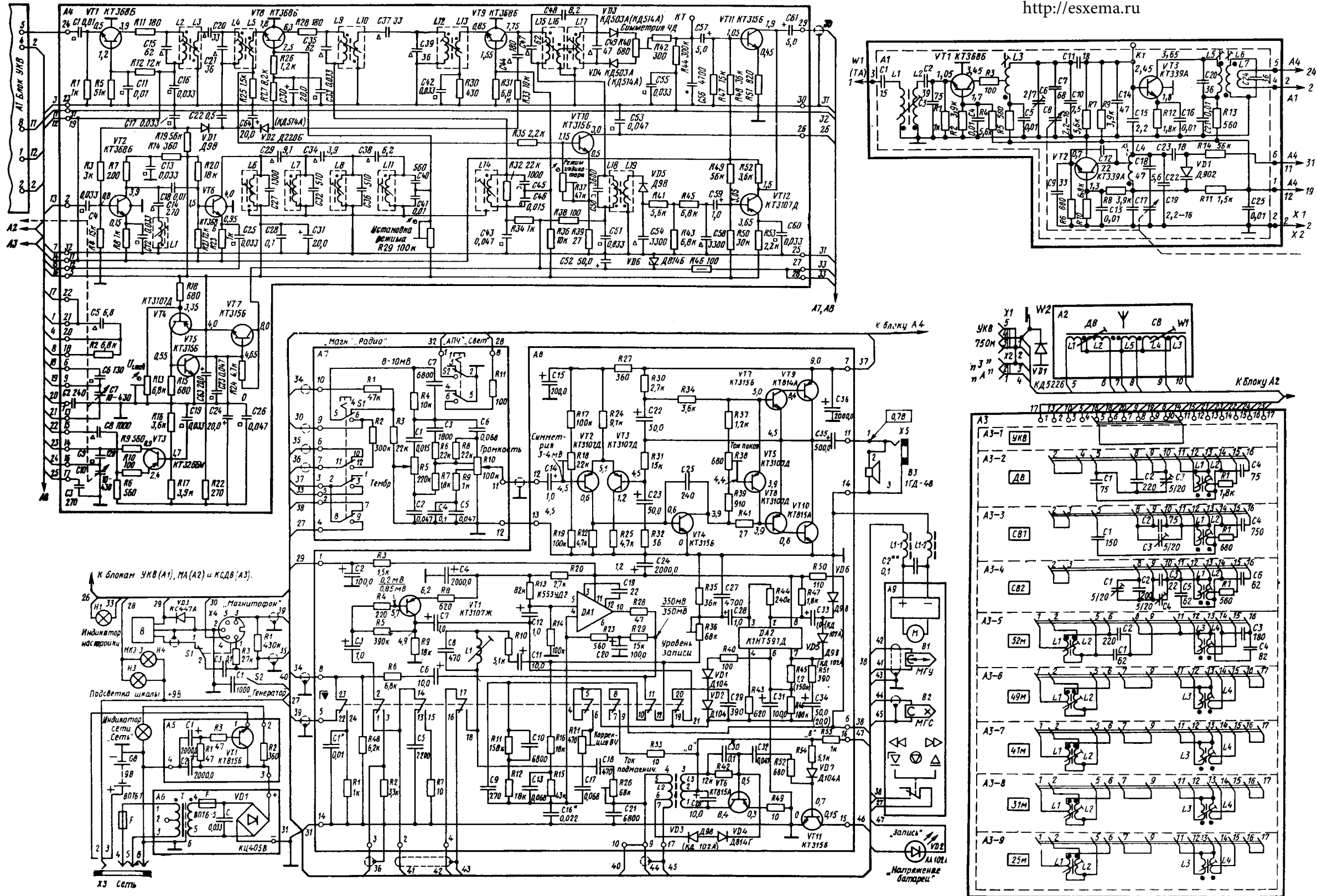
Принципиальная электрическая схема магнитофона "ВЭФ-260"
