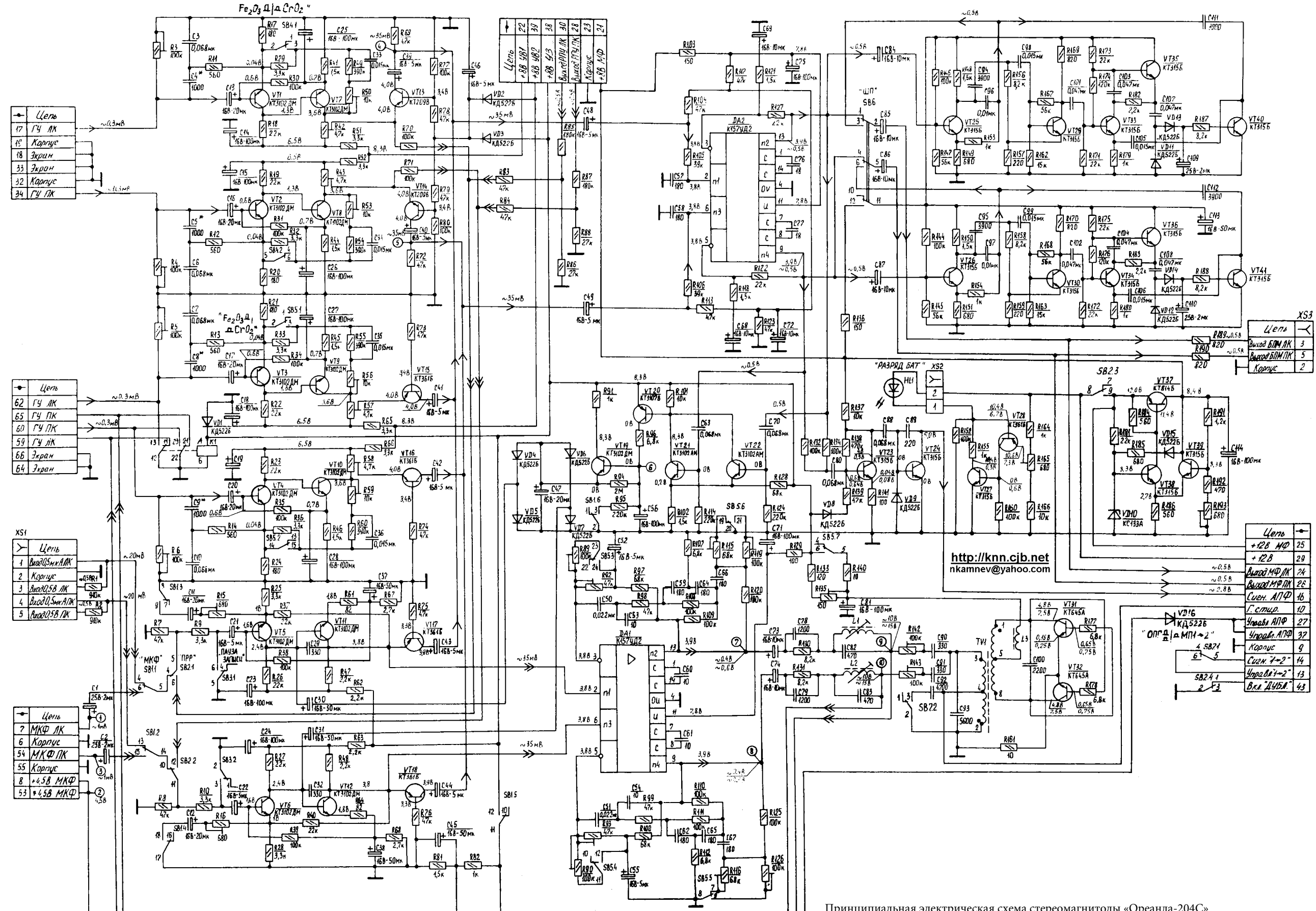
Принципиальная электрическая схема стереомангитолы «Оранда-204С»
