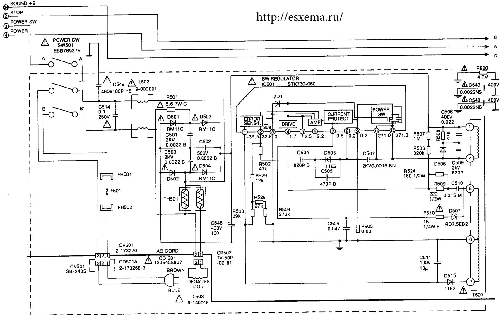
Принципиальная схема блока преобразователя питания телевизора АТЕС TV 1402МК9
