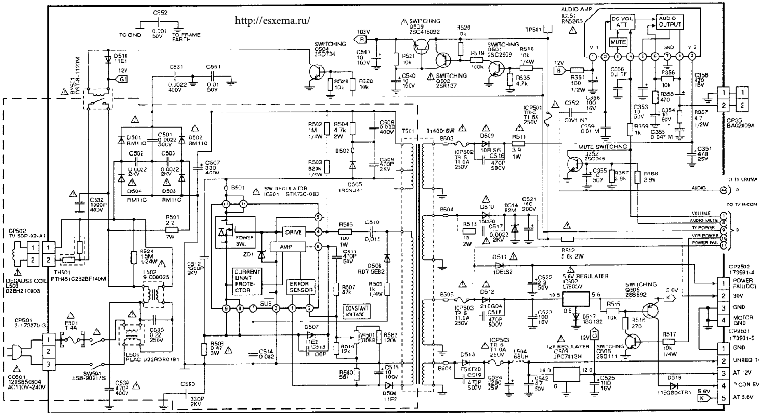
Схема блока питания телевизора AIWA VX-T2020
