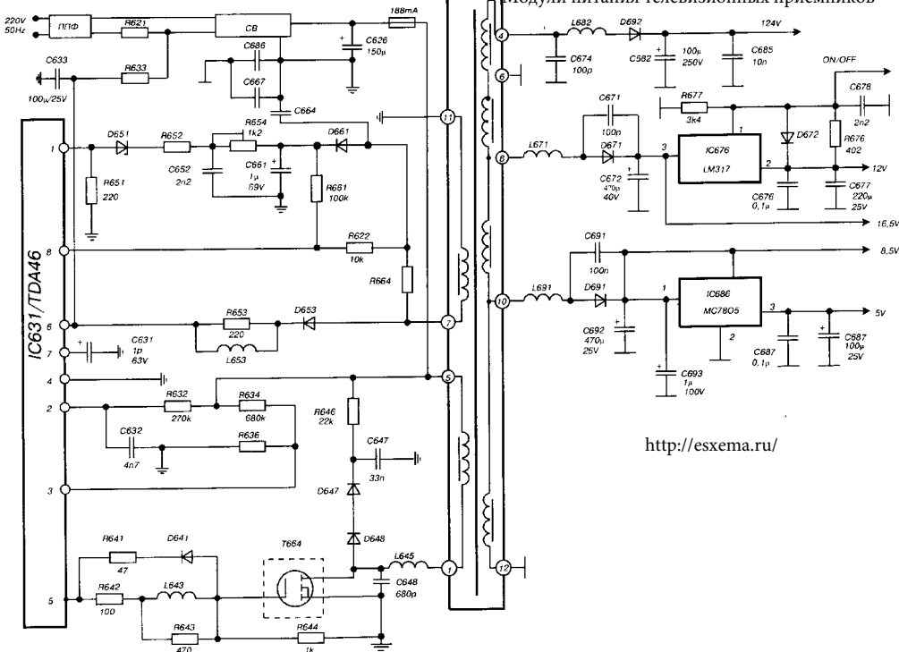
Электрическая схема импульсного БП (блок питания) телевизора «GRUNDIG» CUC4400
