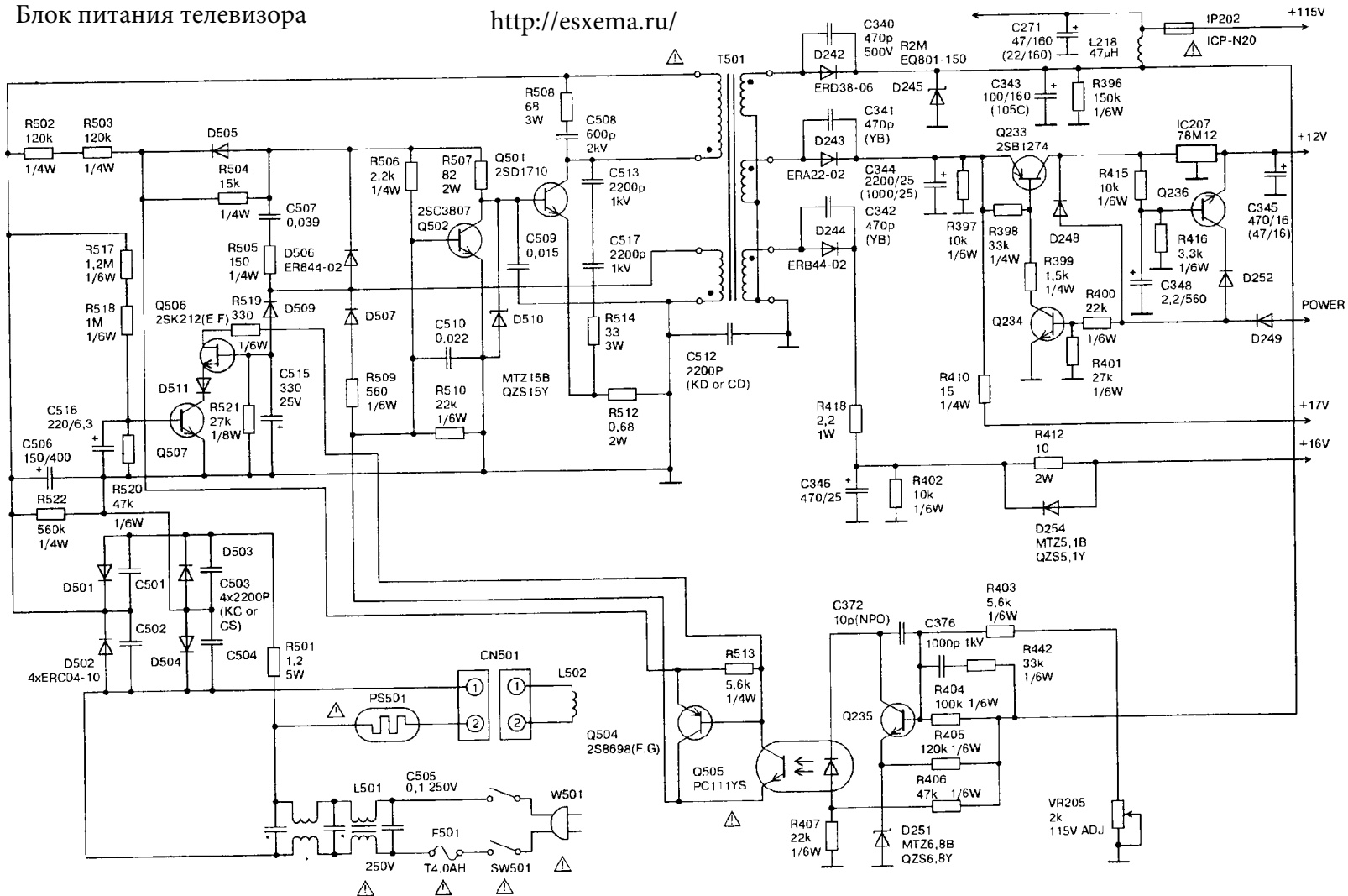
Схема источника питания для телевизора FUNAI моделей TV-2000 MK7, TV-2008 GL
