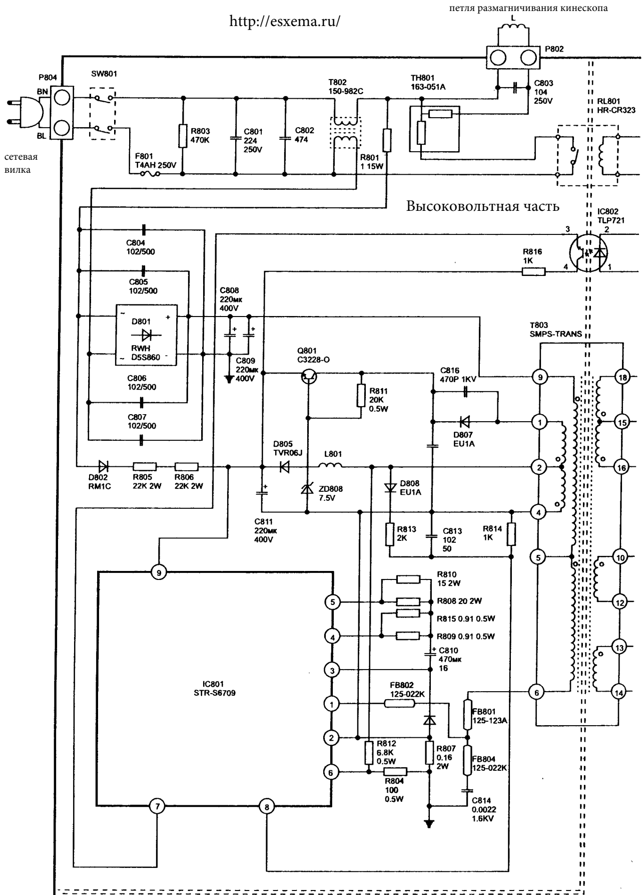
Блок питания телевизора «GOLDSTAR» CF-25/29C36
