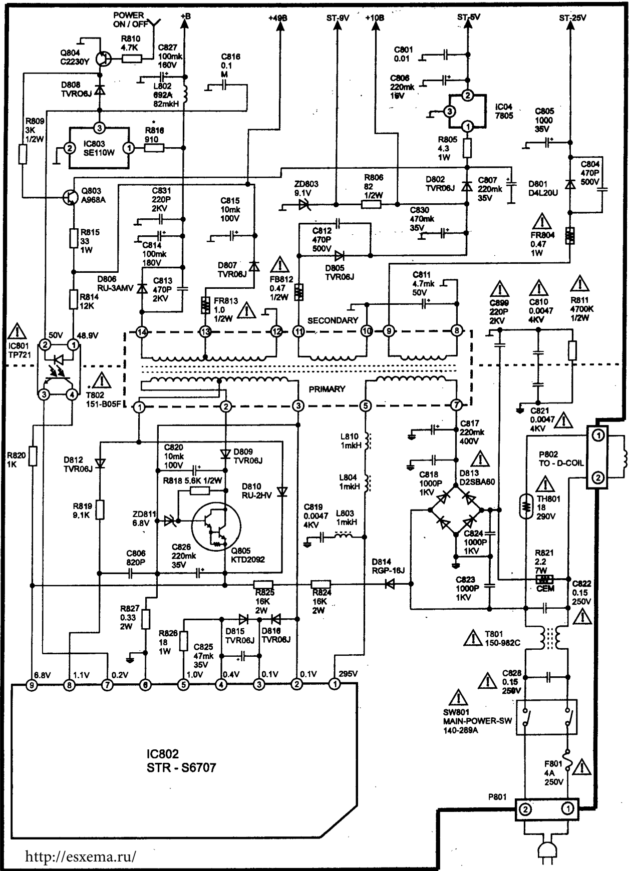
Блок питания импульсного типа "GOLDSTAR" (LG) CF-20E20B, CF-21E20B, CF-21D10Y
