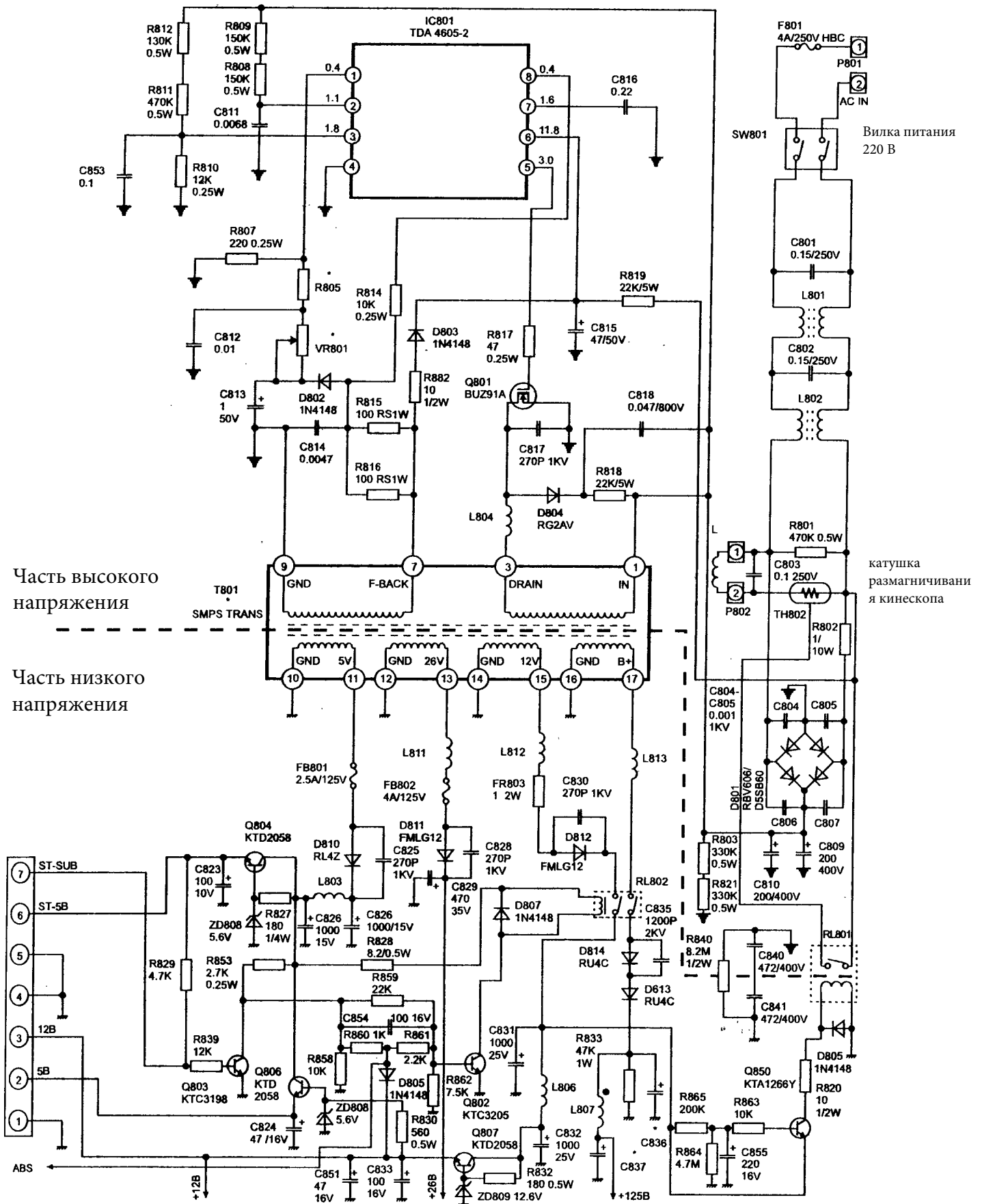
Схема источника питания телевизоров «GOLDSTAR» CF29C20J, CF25C32J, CF29C32J (шасси PC33J)
